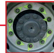
DANGER! wheelnut have loosened Montage à risque
